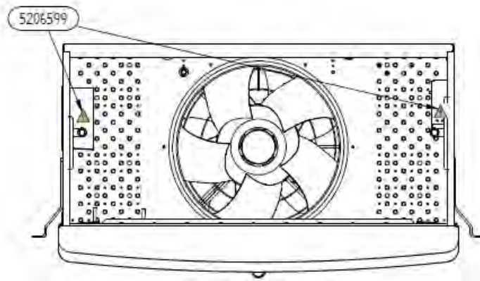
Ansicht Lufteintrittsseite hinter dem Berührungsschutzgitter
